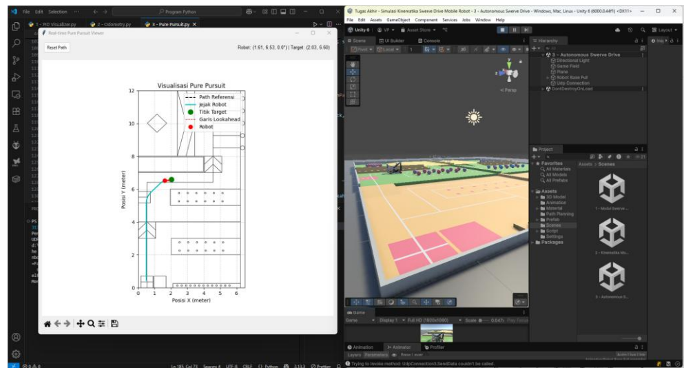
Gambar 3. Simulasi Navigasi Otonom Pure Pursuit
